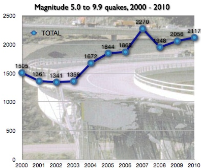
Рис. 4. График количества землетрясений с магнитудой 5 баллов и выше за последнее десятилетие. В 2011 году количество землетрясений с магнитудой от 5 баллов перевалило за 2800... сайт American Daily Herald
