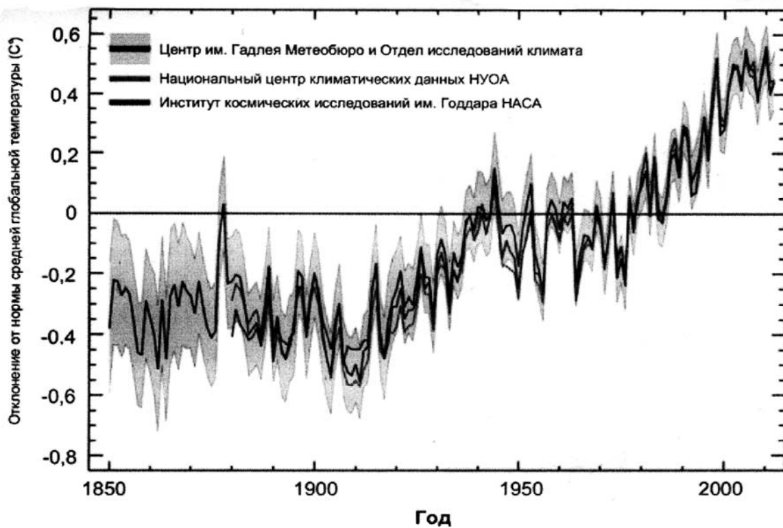
Рис. 3. Температурные вариации с 1850 по 2010 годы.
